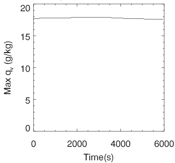
vapor, 15km bubble
